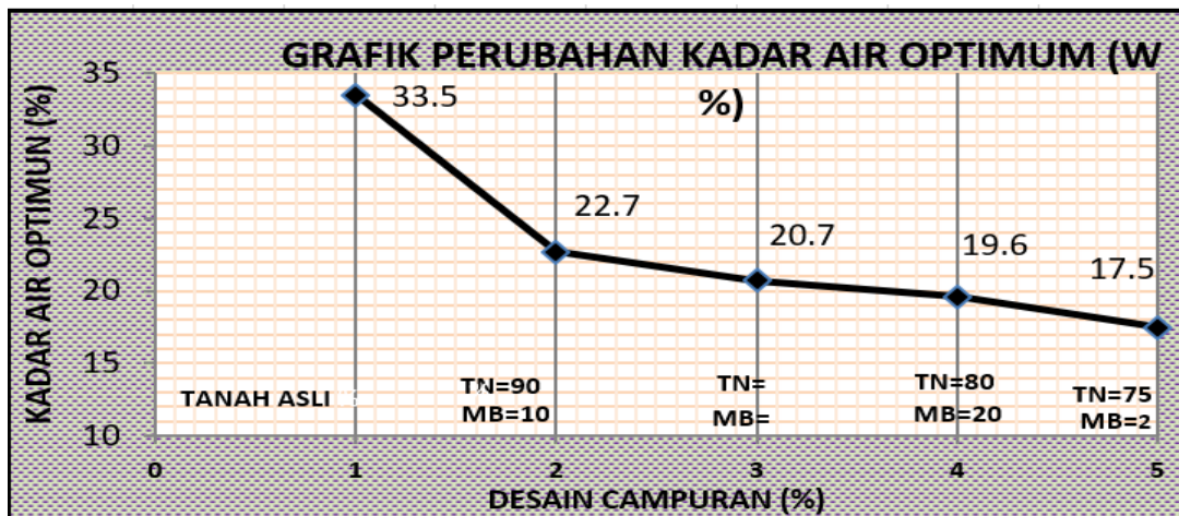
Gambar 4. 19 Grafik Proctor Standart yang menunjukkan contoh Tanah Asli yang mengandung campuran Mortar Busa.
