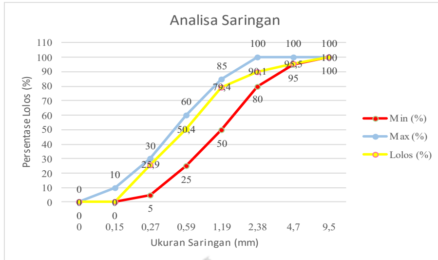
Gambar 4.1. Grafik analisa saringan
