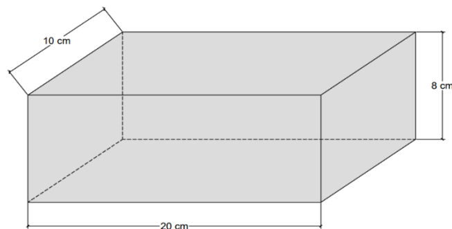
Gambar 3.2. Ukuran sampel kuat lentur
