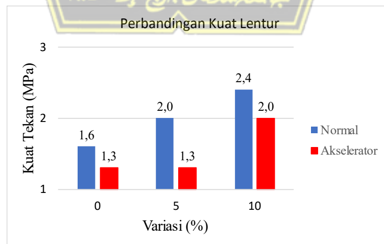
Gambar 4.5. Grafik perbandingan kuat lentur
