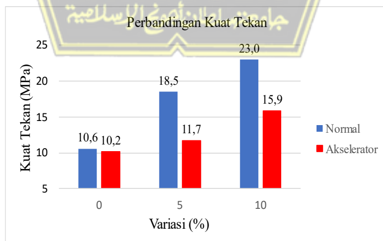
Gambar 4.4. Grafik perbandingan kuat tekan
