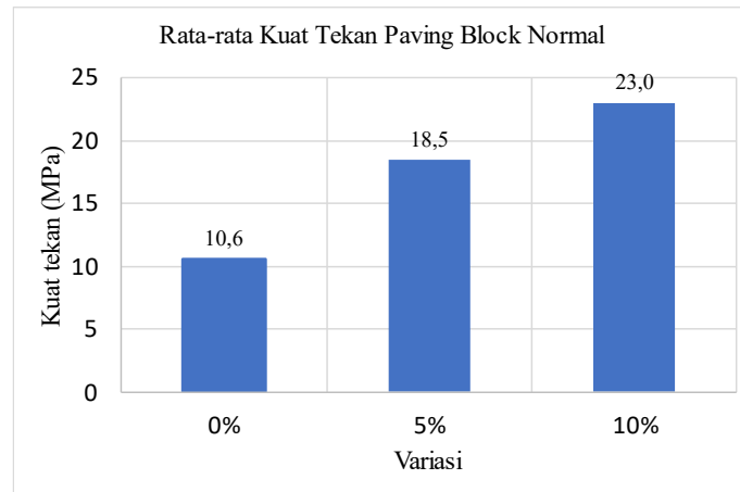
Gambar 4.2. Grafik rata-rata kuat tekan paving block normal
