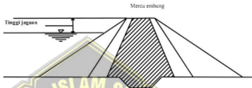
Gambar 2.2. Tinggi Jagaan (Sumber: Kriteria Desain Embung , 1994)
