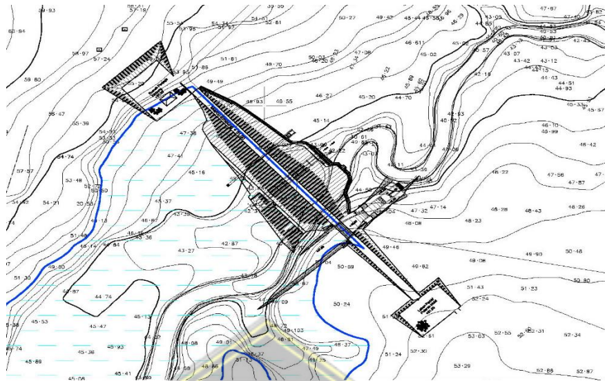
Gambar 2.3. Desain Embung Kaliombo
