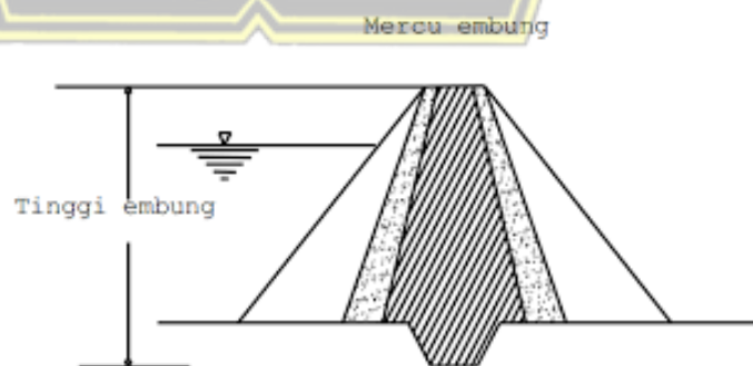
Gambar 2.1 Tinggi embung (Sumber: Kriteria Desain Embung, 1994)
