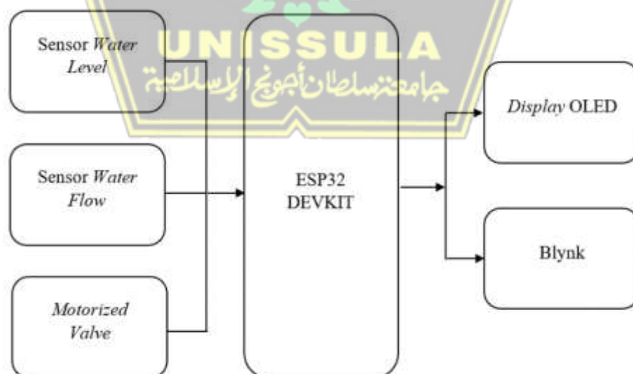
Gambar 3.1 Diagram Blok Usulan Desain 1
