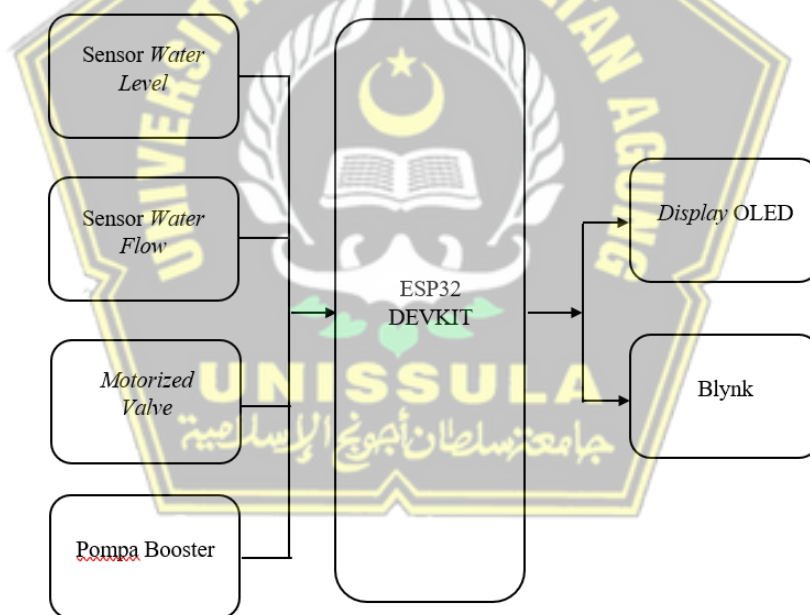
Gambar 3.6 Diagram Blok Usulan Desain 2
