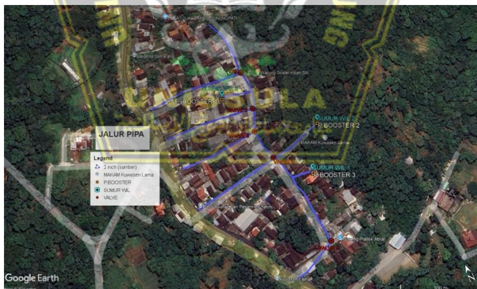
Gambar 3.9 Desain Simulasi Usulan Kedua Dengan Pengaturan Valve & penambahan Pompa Booster
