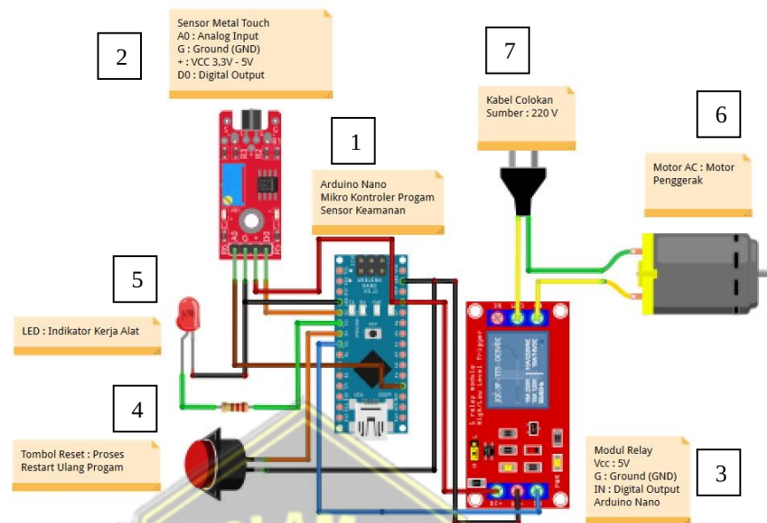
Gambar 3. 4 Desain rangkaian sistem
