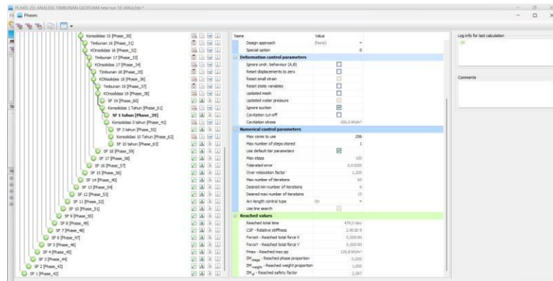
Gambar 4.24 Nilai SF Pada Konsolidasi Timbunan 1 Tahun
