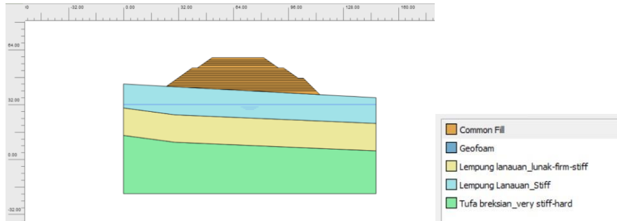
Gambar 4.7 Permodelan Tanah Timbunan Tanpa Perkuatan
