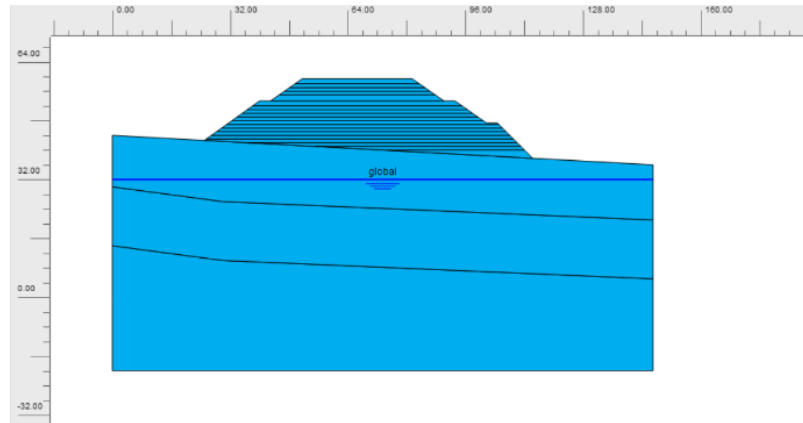
Gambar 4.14 Permodelan Muka Air Tanah
