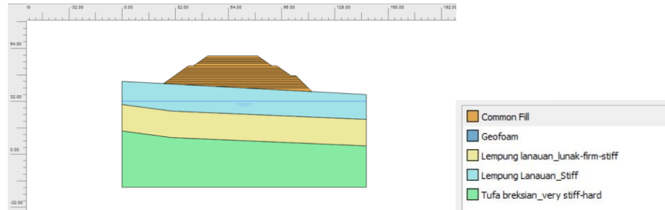
Gambar 4.12 Permodelan Tanah Timbunan Tanpa Perkuatan
