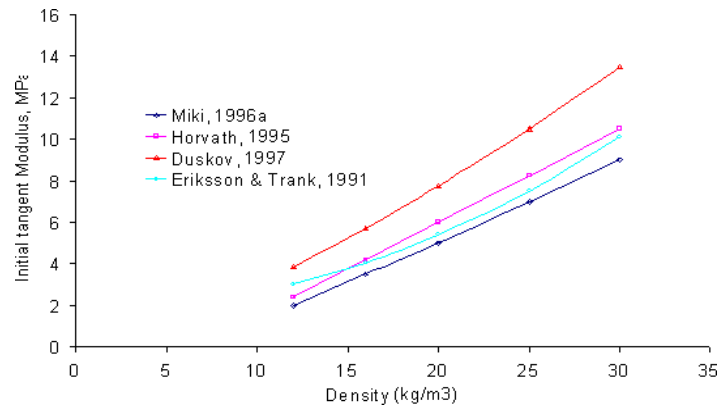
Gambar 2.5 Grafik Modulus tangen awal untuk EPS Geofoam (Dus-kov, 1997 dan Eriksson dan Trank, 1991)
