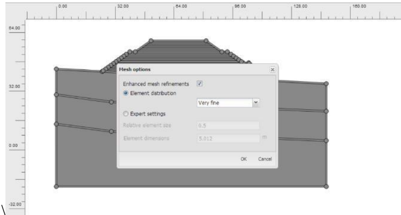
Gambar 4.9 Jendela Mesh
