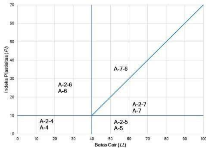
Gambar 2.1 Rentang batas cair (LL) dan indeks plastisitas (PI) untuk tanah yang masuk dalam kelompok A-2, A-4, A-5, A-6, dan A-7 (AASHTO M145 atau ASTM D3282)
