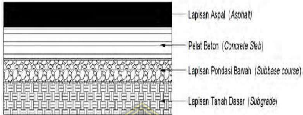
Gambar 2.10 Struktur Perkerasan Komposit Anas (2004)
