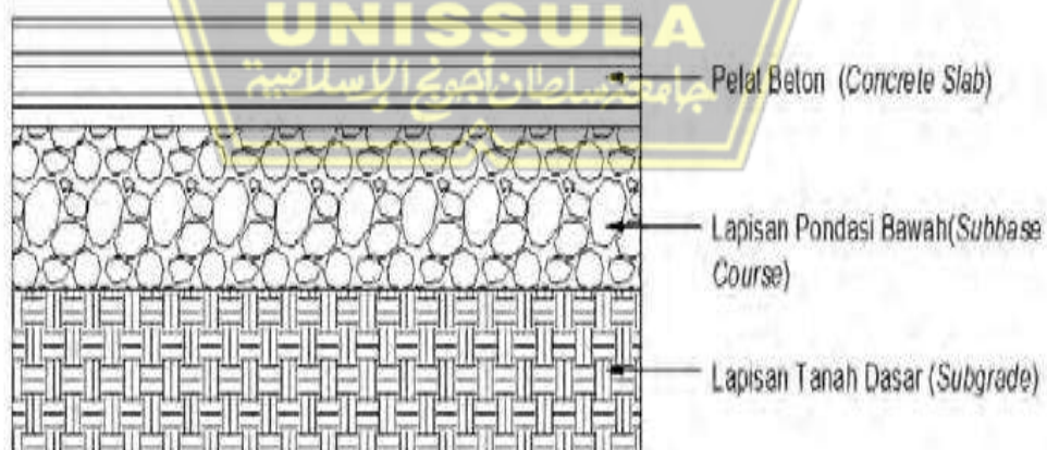
Gambar 2.9 Struktur Perkerasan kaku Anas (2004)
