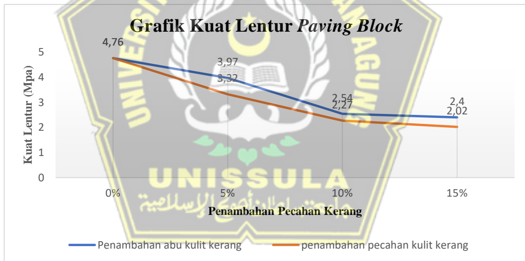
Gambar 4.14 Grafik Kuat lentur Paving Block Penambahan Abu Kulit Kerang Dan Pecahan Kulit Krang hijau.
