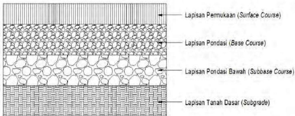
Gambar 2.8 Struktur Perkerasan Lentur Anas (2004)
