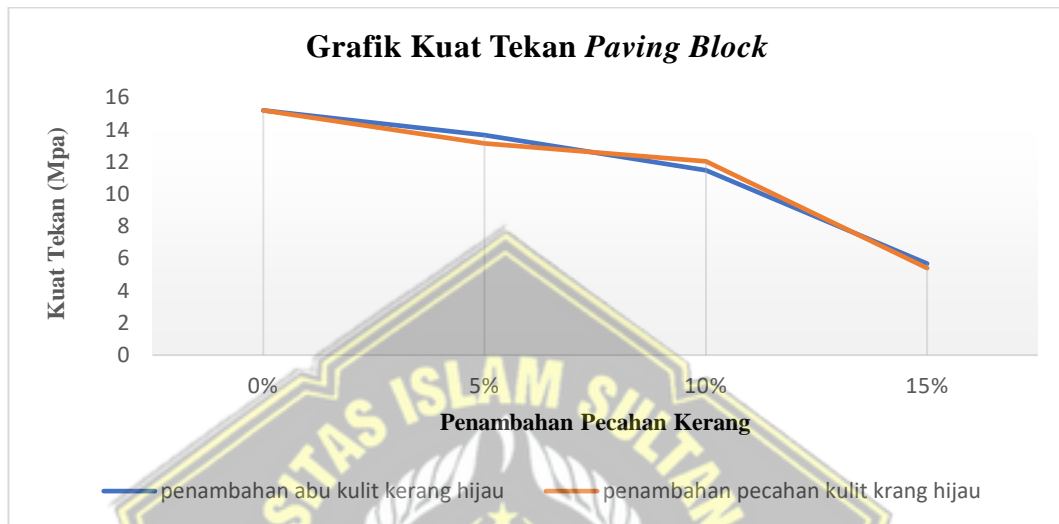
Gambar 4.11 Grafik Kuat Tekan Paving Block Penambahan Abu Kulit Kerang Dan Pecahan Kulit Krang hijau.
