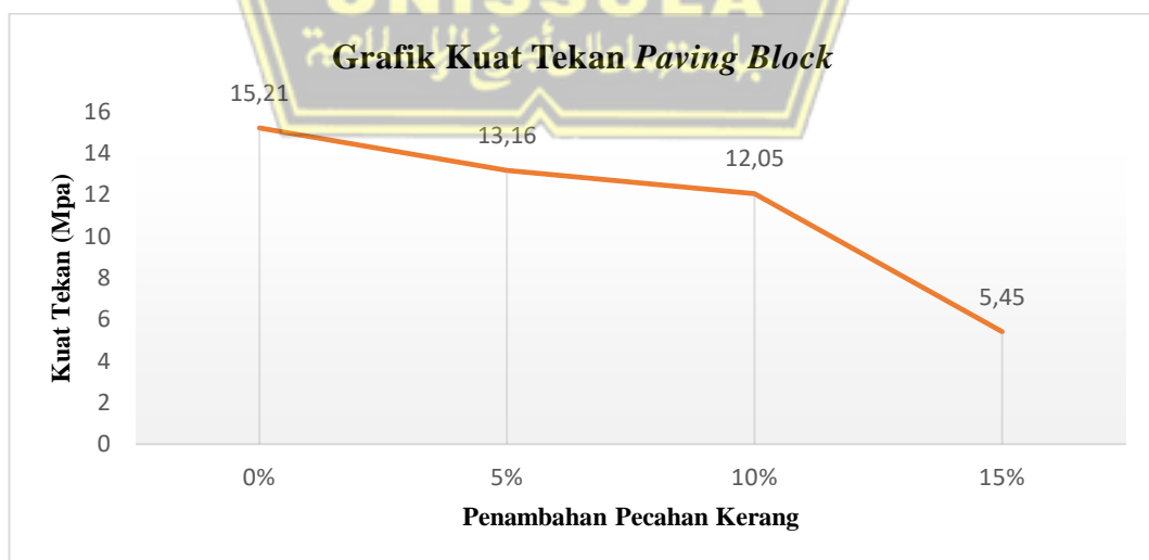
Gambar 4.10 Grafik Kuat Tekan Paving Block Penambahan pecahan kulit Kerang Hijau.
