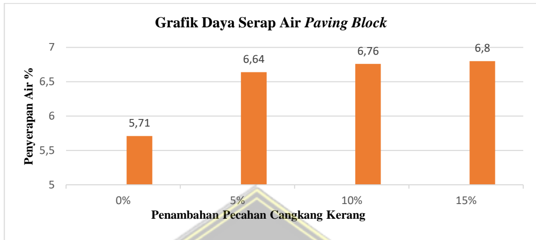
Gambar 4.7 Grafik Pengukuran Daya Serap Air Paving Block Dengan Penambahan pecahan Cangkang Kerang hijau
