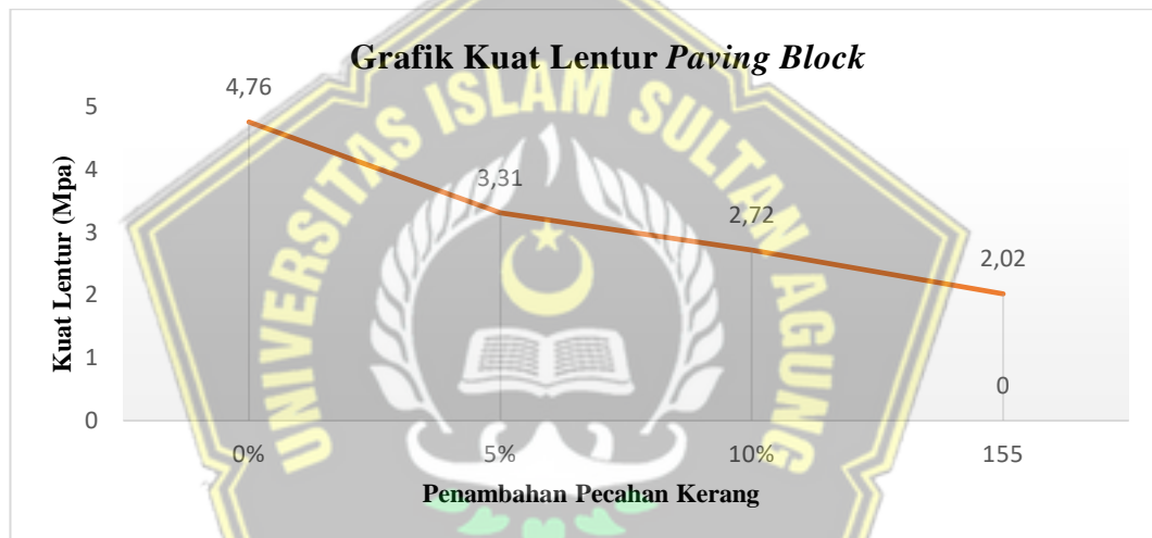
Gambar 4.13 Grafik Kuat Lentur Paving Block Penambahan Abu Kulit Kerang.
