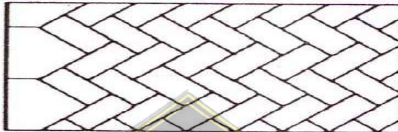
Gambar 2.19 Tulang Ikan 45° Penguncian Paling Baik
