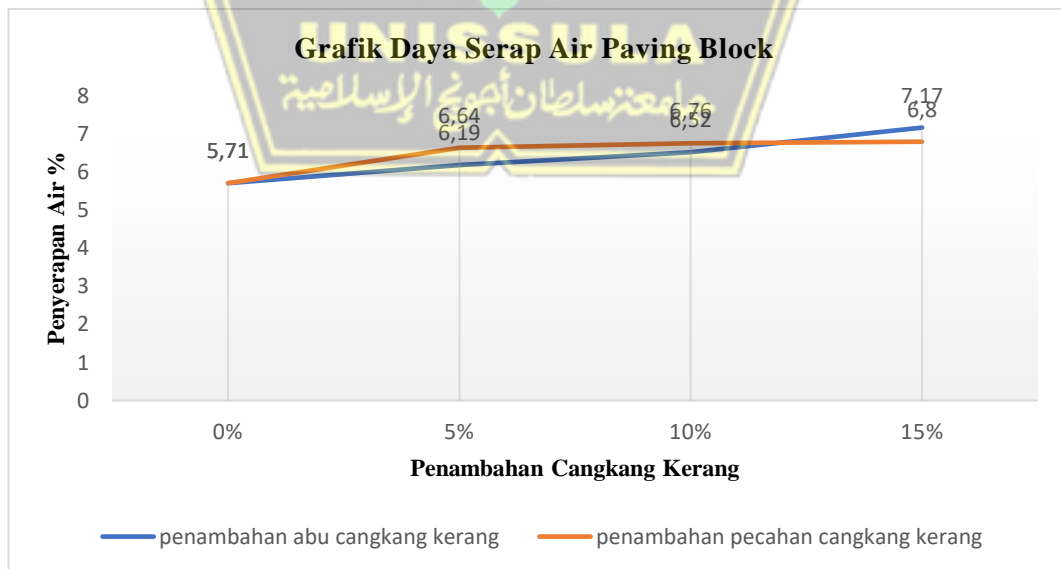
Gambar 4.8 Grafik Rekapitulasi Daya Serap Air Paving Block Dengan Penambahan Abu Kulit Kerang Dan Pecahan Kulit Krang hijau.
