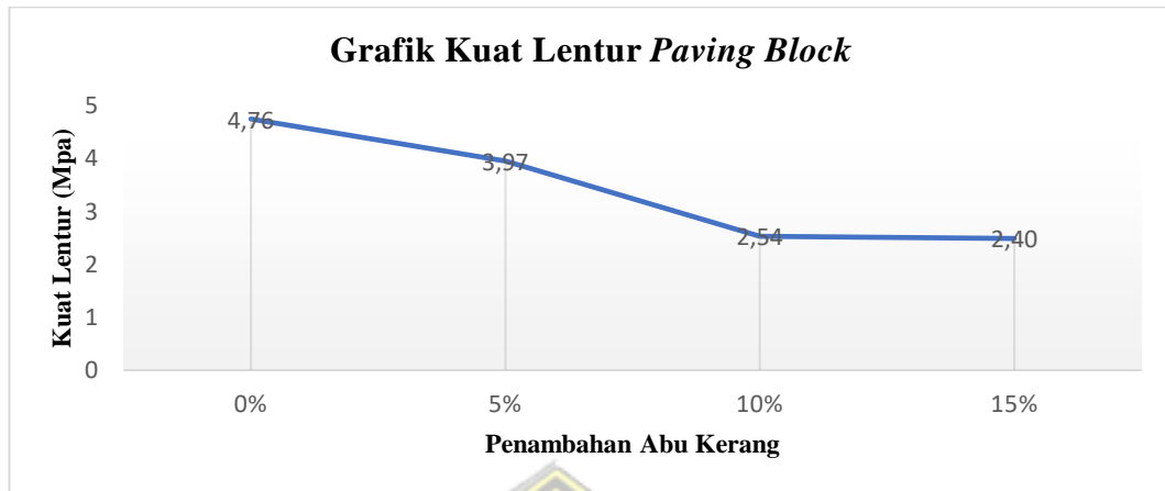
Gambar 4.12 Grafik Kuat Lentur Paving Block Penambahan Abu Kulit Kerang.
