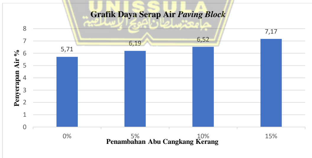
Gambar 4.6 Grafik Pengukuran Daya Serap Air Paving Block Dengan Penambahan Abu Cangkang Kerang hijau.
