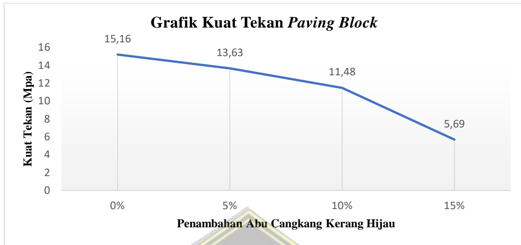
Gambar 4.9 Grafik Kuat Tekan Paving Block Penambahan Abu kulit Kerang Hijau.
