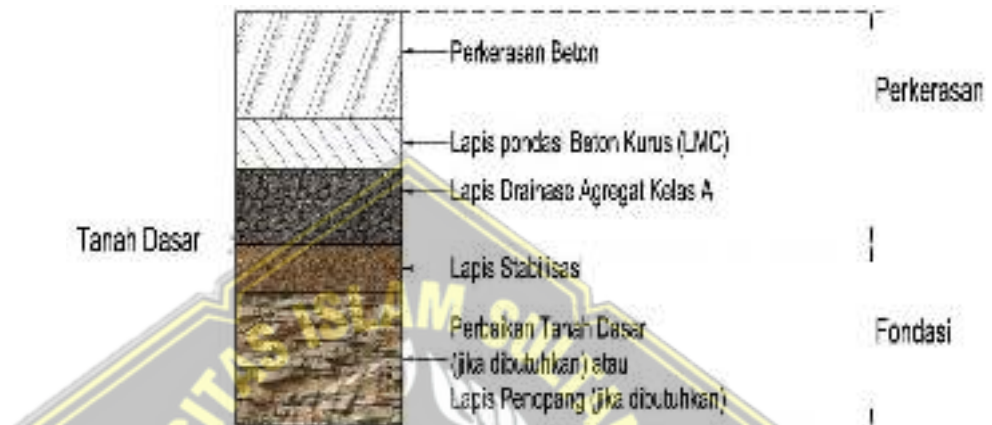
Gambar 2. 2 Potongan melintang perkerasan jalan kaku (Beton) No. 02/M/BM/2017 adalah sebagai berikut :
