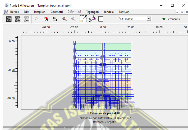
Gambar 4.23 Tampilan Tekanan Air Pori
