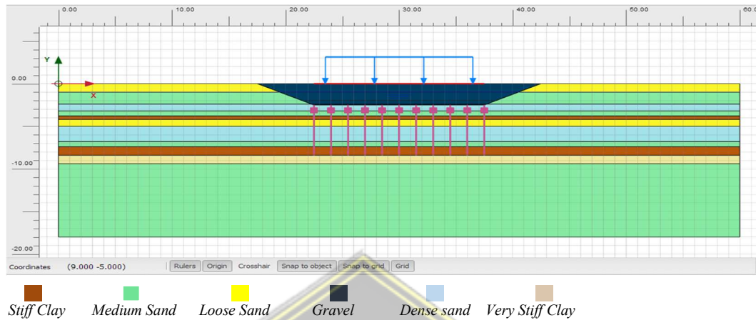
Gambar 4.16 Pemodelan Rigid Inclution pada tanah asli
