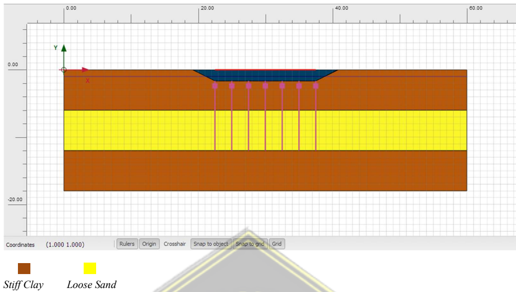
Gambar 4.12 Pemodelan Rigid Inclusion
