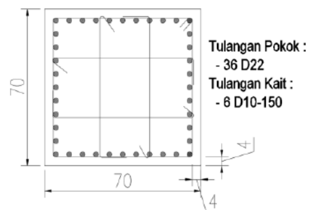
Gambar 4. 41. Tulangan Tengah Kolom K1
