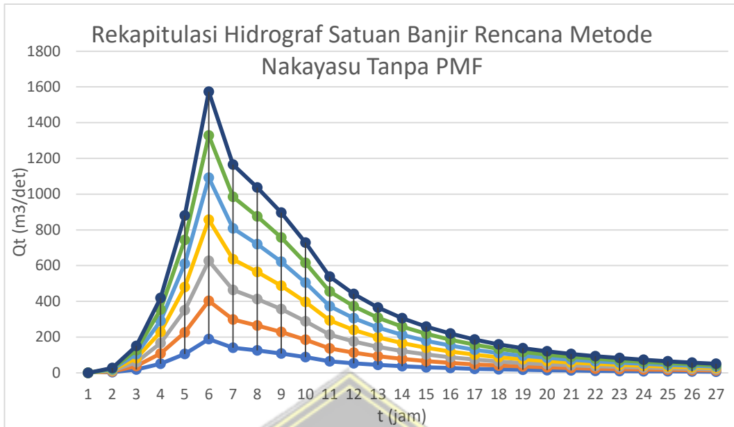
Gambar 4.7. Grafik Rekapitulasi Hidrograf Satuan Banjir Rencana Metode Nakayasu tanpa PMF
