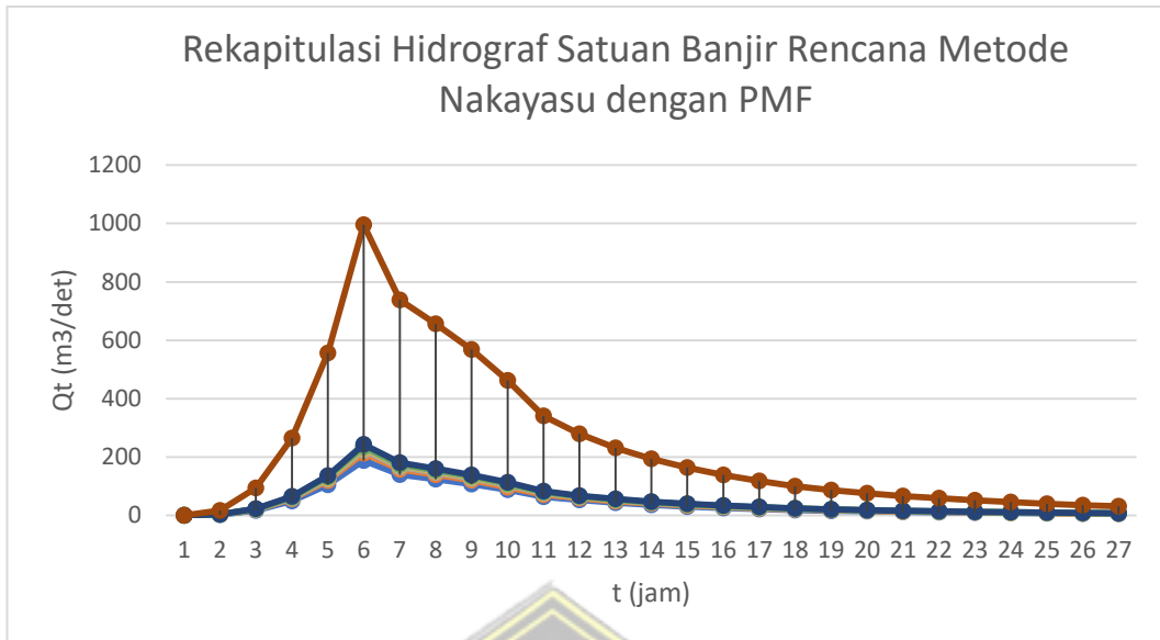
Gambar 4.6. Grafik Rekapitulasi Hidrograf Satuan Banjir Rencana Metode Nakayasu dengan PMF
