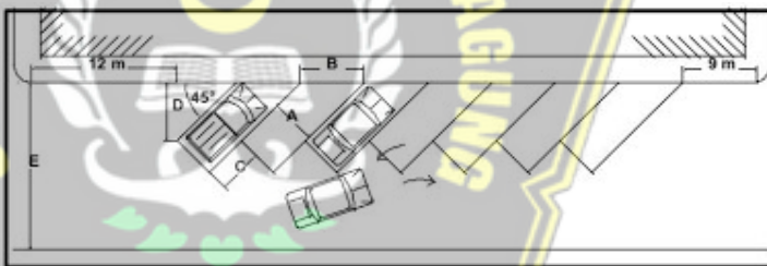
Gambar 2.8. Pola Parkir Bersudut 45^\circ
