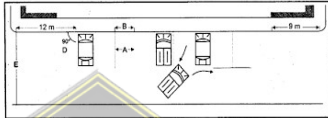
Gambar 2.10. Pola Parkir Tegak Lurus 90°
