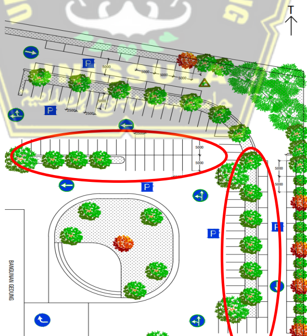
Gambar 4.9. Pola Parkir Tegak Lurus di Rumah Sakit Islam Sultan Agung (sumber : gambar AutoCAD pribadi )
