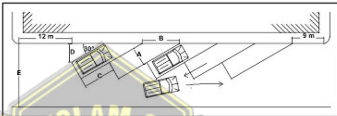
Gambar 2.7. Pola Parkir Bersudut 30^\circ
