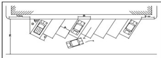
Gambar 2.9. Pola Parkir Bersudut 60^\circ
