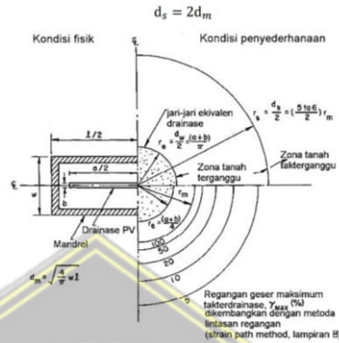
Gambar 2.19 Prediksi Zona Pengaruh di Sekitar Mandrel
