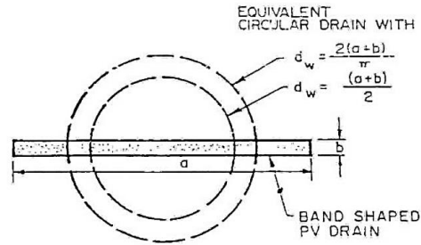
Gambar 2.18 Transformasi Penampang Diameter Setara PVD
