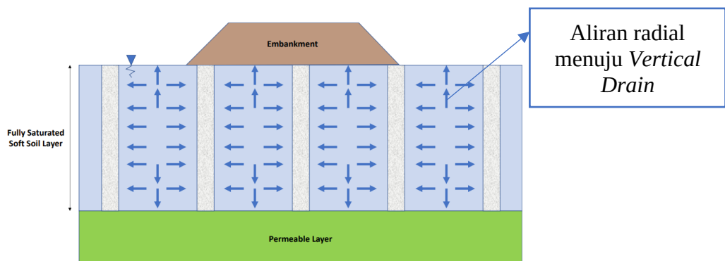
Gambar 2.12 Jalur Drainase Selama Proses Konsolidasi dengan PVD
