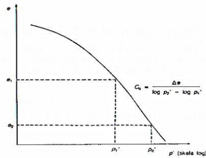
Gambar 2.3 Indeks Pemampatan (Hardiyatmo, 2003)
