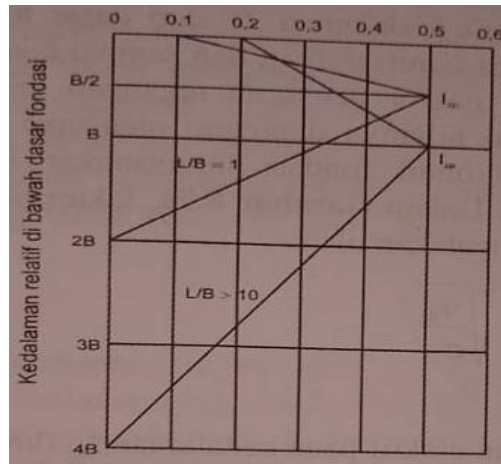
Gambar 2.8 Grafik Faktor Pengaruh Regangan untuk Pondasi Kaku Iz (Hardiyatmo, 2014)
