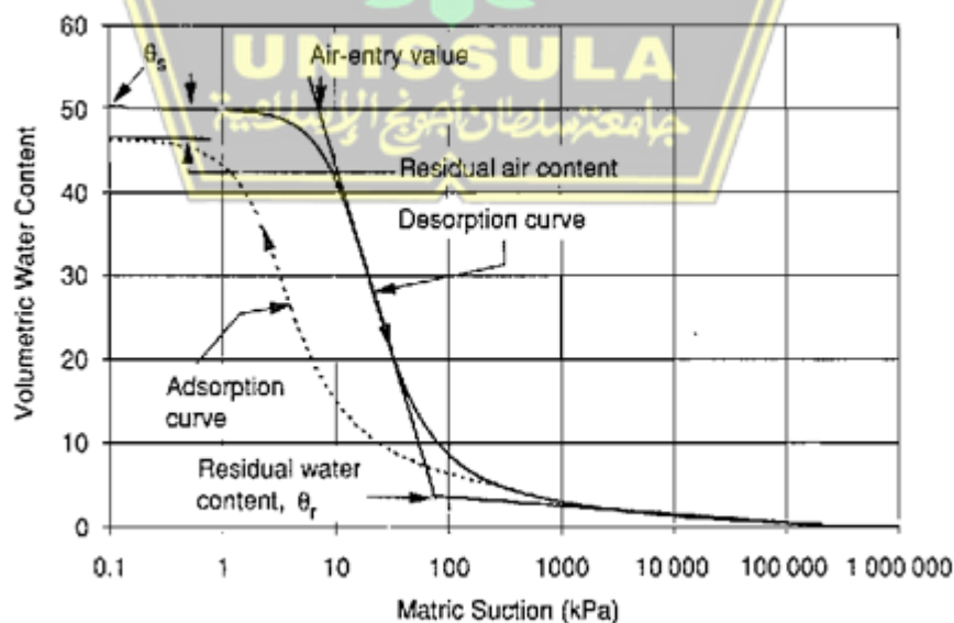
Gambar 2. 1 Definisi variabel-variabel yang terdapat pada soil-water
