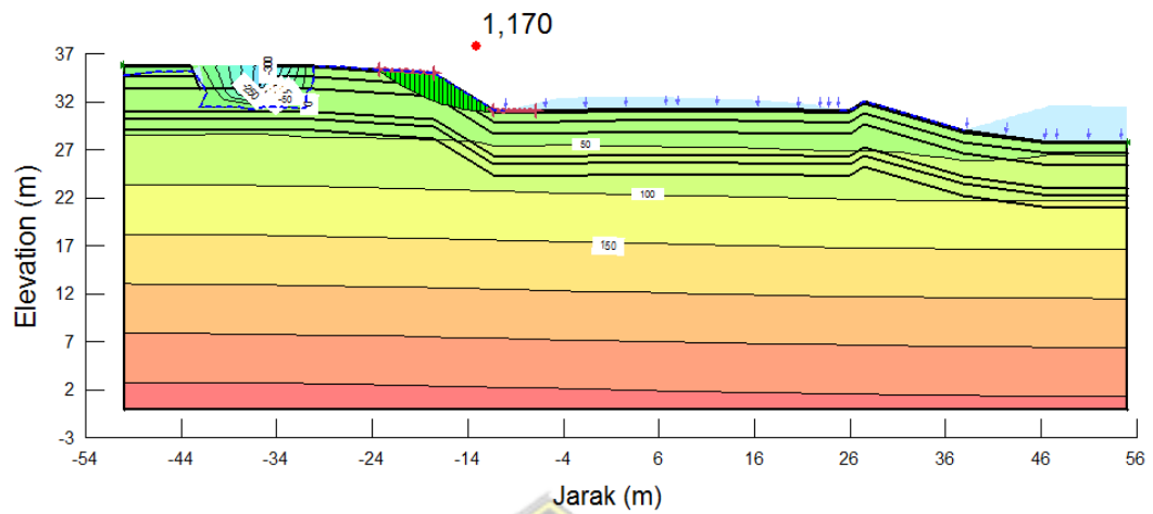
Gambar 4. 50 Nilai SF Curah Hujan Periode 100 tahun
