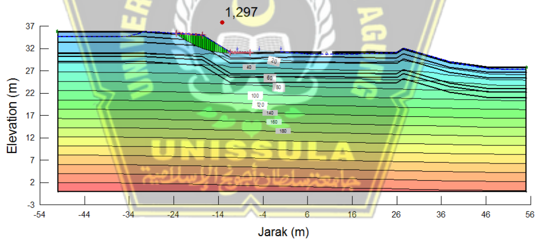
Gambar 4. 37 Nilai SF Curah Hujan Periode 2 tahun
