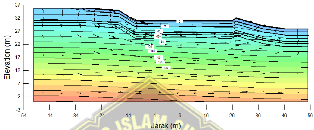
Gambar 4. 28 kontur Pressure Head pada permodelan awal
