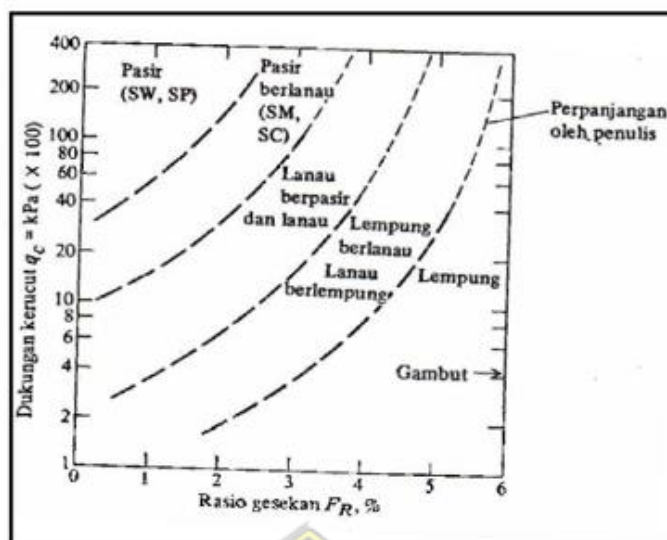
Gambar 4. 7 Klasifikasi Tanah Grafik Hubungan q_c dan R_f Menurut Robertson dan Campanella (Bowles, 1997)
