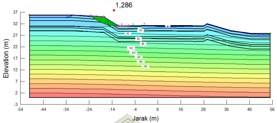
Gambar 4. 42 Nilai SF Curah Hujan Periode 100 tahun
