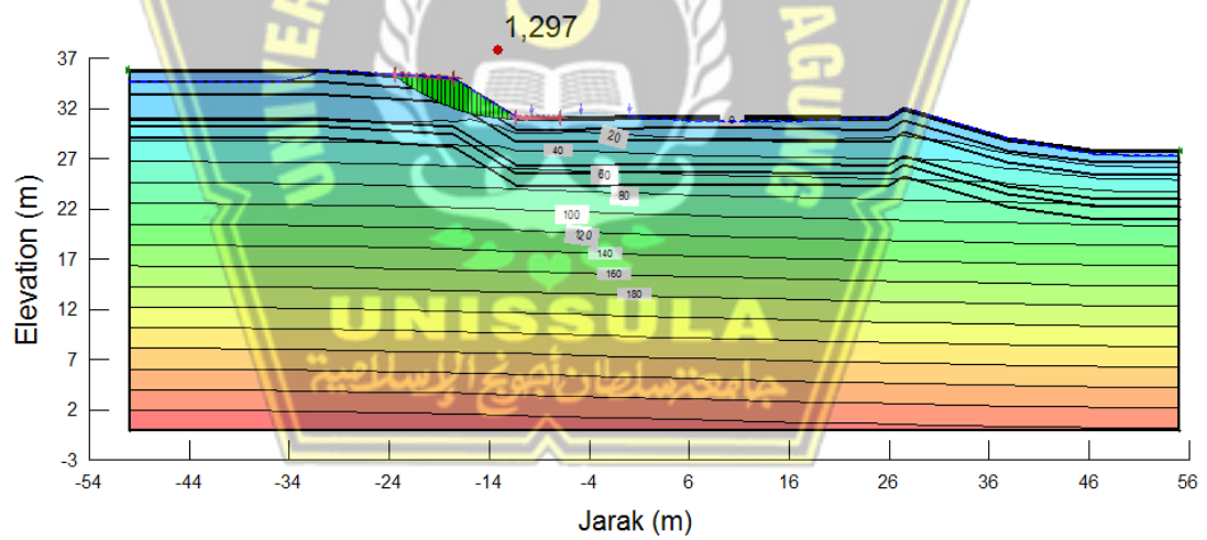
Gambar 4. 39 Nilai SF Curah Hujan Periode 10 tahun
