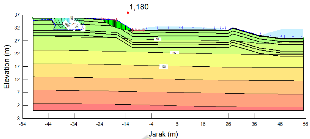
Gambar 4. 46 Nilai SF Curah Hujan Periode 5 tahun
