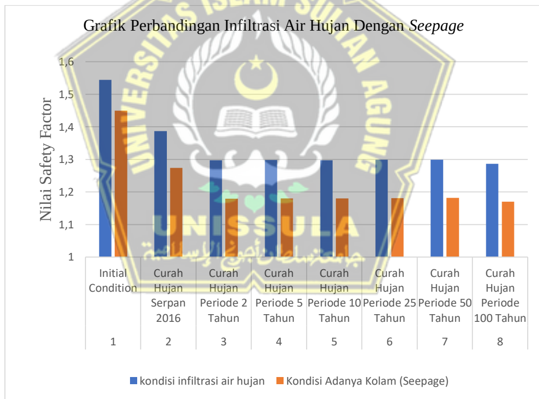
Gambar 4. 58 Grafik Perbandingan Infiltrasi Air Hujan Dengan Rembesan ( Seepage )
