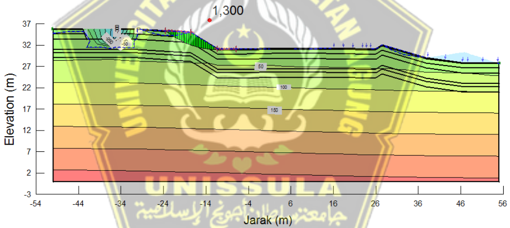
Gambar 4. 55 Nilai SF Curah Hujan Periode 25 tahun
