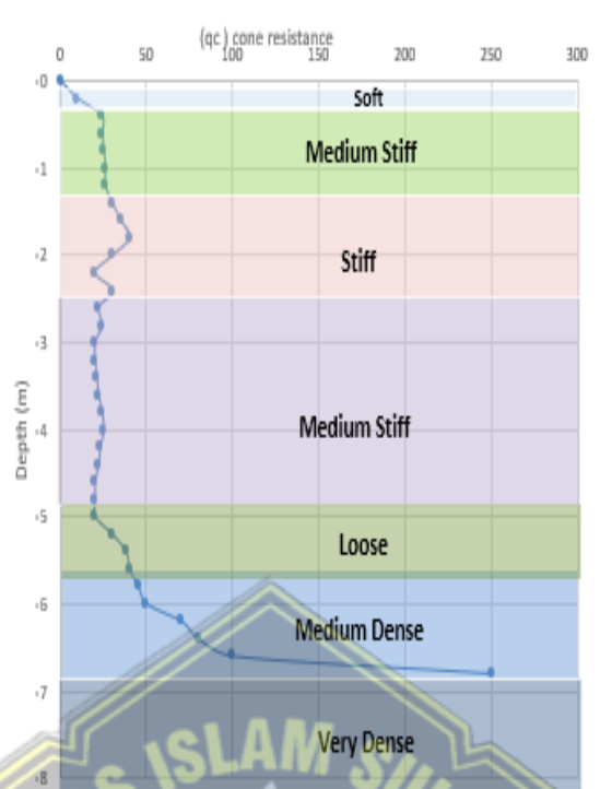
Gambar 4. 8 Grafik Sondir
