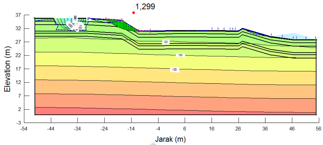
Gambar 4. 54 Nilai SF Curah Hujan Periode 10 tahun
