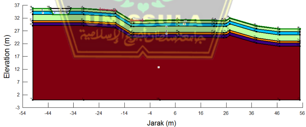
Gambar 4. 33 Permodelan SLOPE/W dengan kolam
