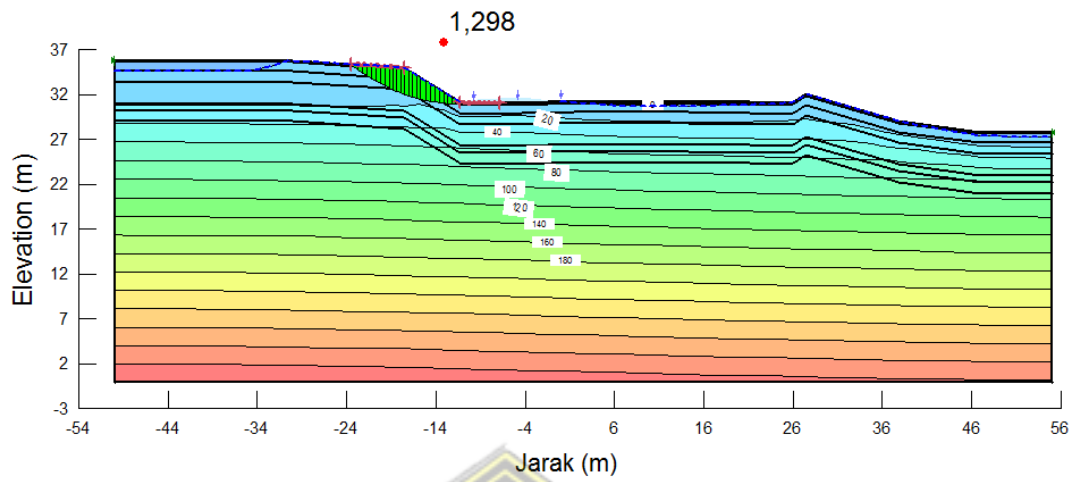
Gambar 4. 38 Nilai SF Curah Hujan Periode 5 tahun
