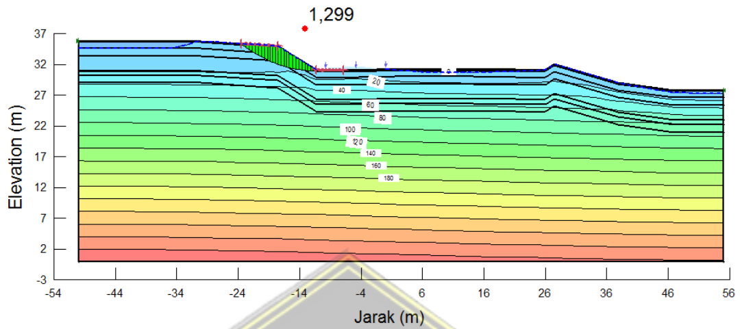
Gambar 4. 40 Nilai SF Curah Hujan Periode 25 tahun
