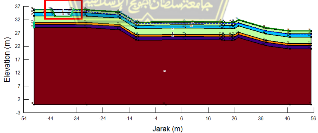
Gambar 4. 21 Permodelan Initial Condition Dengan Kolam (Seepage)
