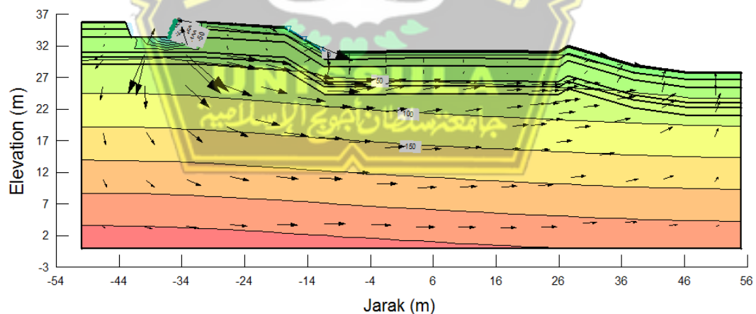
Gambar 4. 29 kontur Pressure Head pada permodelan dengan adanya kolam
