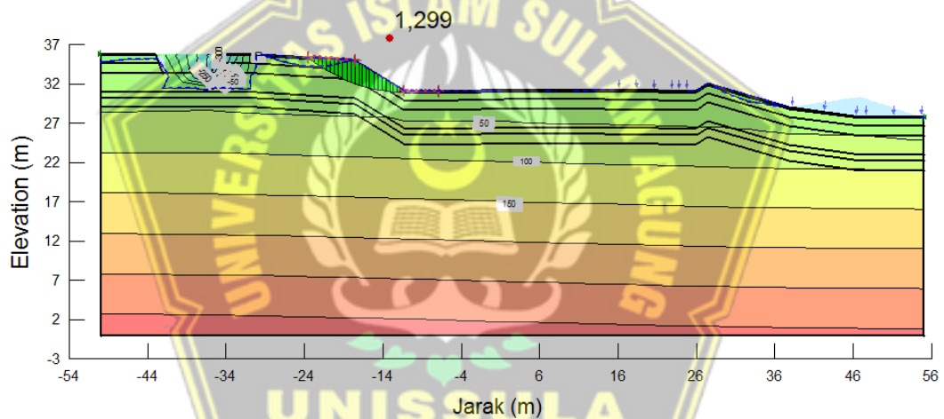
Gambar 4. 53 Nilai SF Curah Hujan Periode 5 tahun
