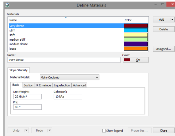
Gambar 4. 34 Input parameter tanah
