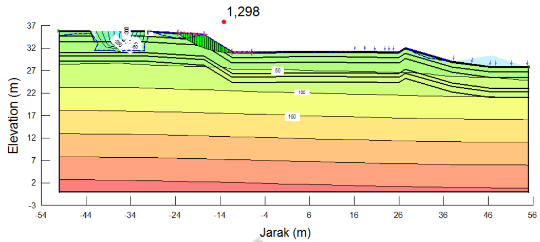
Gambar 4. 52 Nilai SF Curah Hujan Periode 2 tahun
