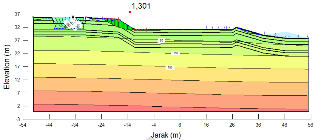
Gambar 4. 56 Nilai SF Curah Hujan Periode 50 tahun
