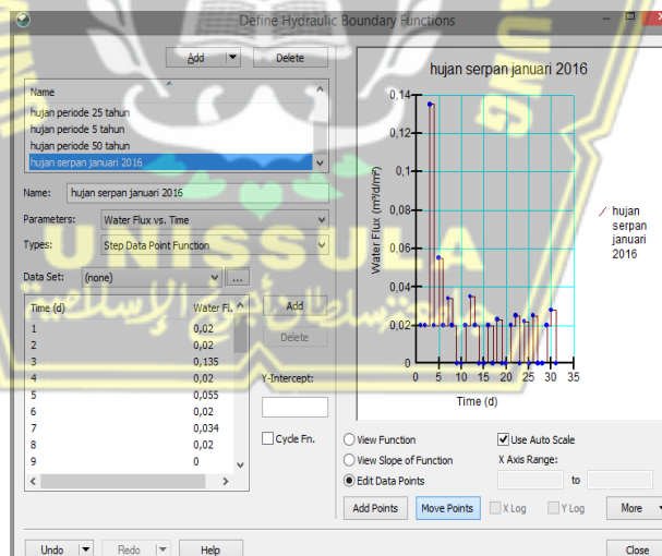
Gambar 4. 23 Data Curah Hujan
