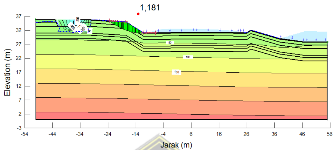
Gambar 4. 48 Nilai SF Curah Hujan Periode 25 tahun
