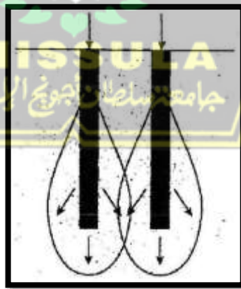
Gambar 2. 5 Tiang Pancang Kelompok
