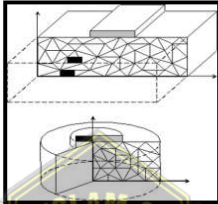
Gambar 2. 12 Contoh Permasalahan Regangan Bidang dan Axi-Simetris
