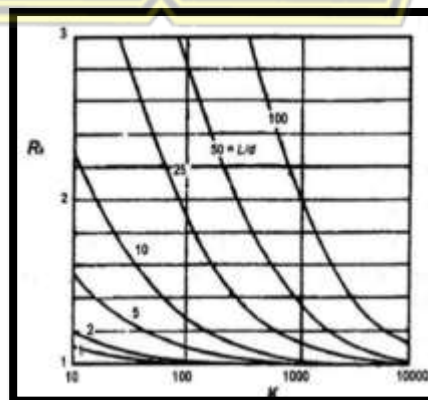
Gambar 2. 7 Faktor Penurunan R_k
