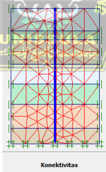
Gambar 4.15 Susunan jaringan elemen ( mesh )
