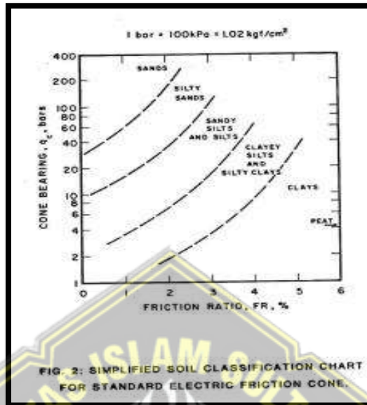
Gambar 2. 1 Grafik Hubungan Tekanan Conus dengan Perlawanan Geser
