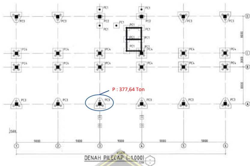
Gambar 4.2 Denah Pilecap Proyek Pembangunan Gedung Teknik Informatika Politeknik Negeri Cilacap
