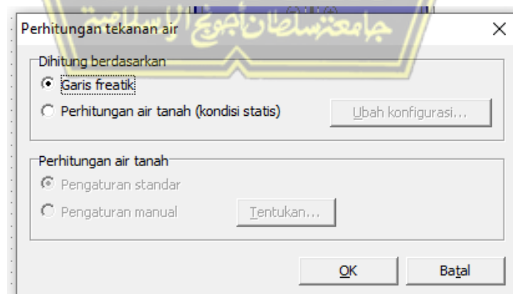
Gambar 4.17 Jendela Perhitungan tekanan air
