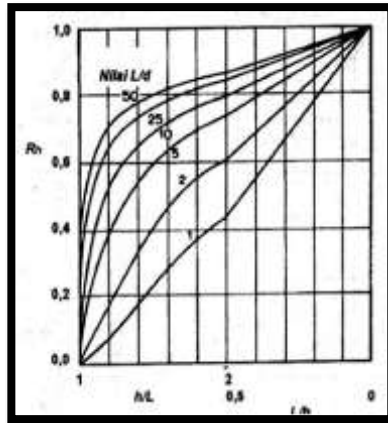
Gambar 2. 8 Faktor Penurunan R_h (Sumber : Poulus dan Davis, 1980)
