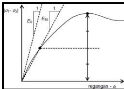
Gambar 2. 13 Contoh Permasalahan Regangan Bidang dan Axi-Simetris
