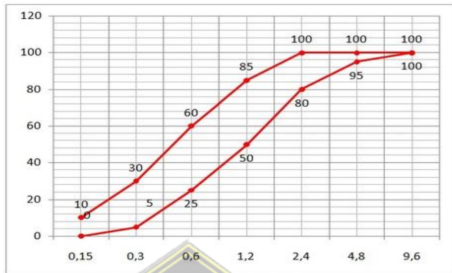
Gambar 2. 2 - Grafik Gradasi Agregat Halus
