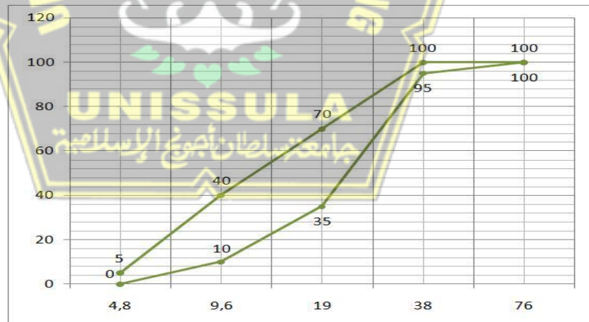
Gambar 2. 1 - Grafik Gradasi Agregat Kasar
