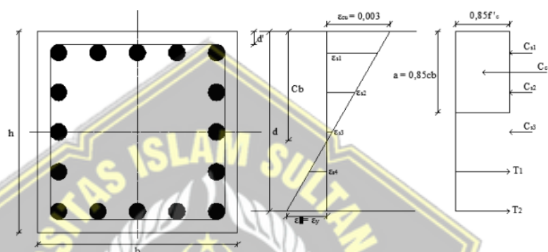
Gambar 2.23 Gambar Kolom Lentur Dua Arah
