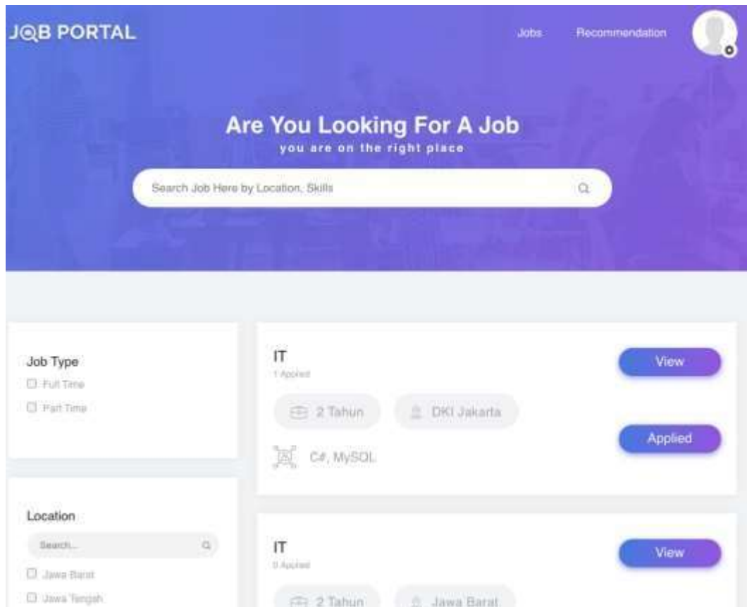
Gambar 4.14: Daftar Lowongan
