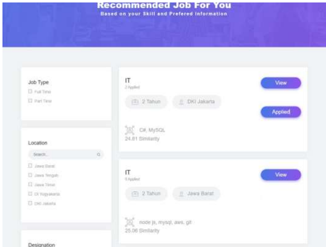
Gambar 4.16: Rekomendasi Lowongan
