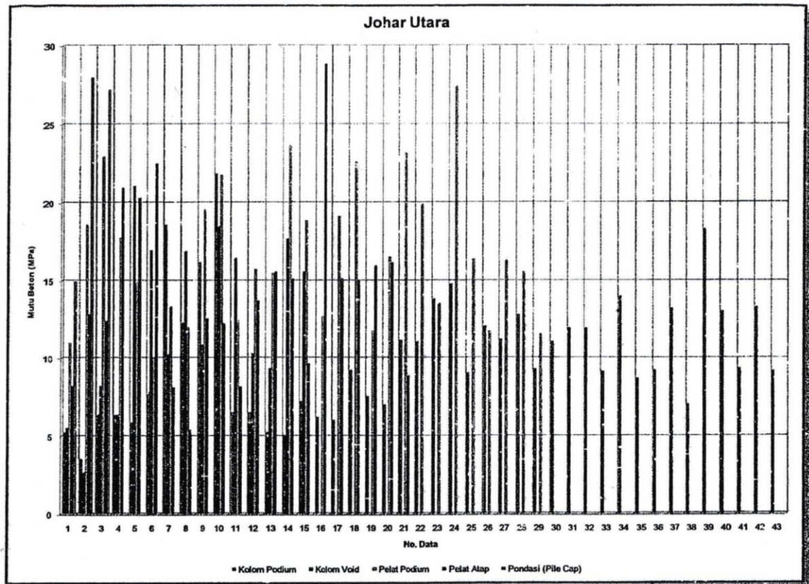
Gambar 22 Kurva kuat tekan sampel beton inti di bangunan Pasar Johar Utara
