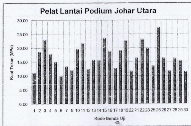
Gambar 19 Kurva sebaran nilai kuat tekan beton pelat lantai podium Pasar Johar Utara
