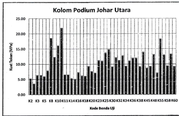
Gambar 17 Kurva sebaran nilai kuat tekan beton kolom podium Pasar Johar Utara
