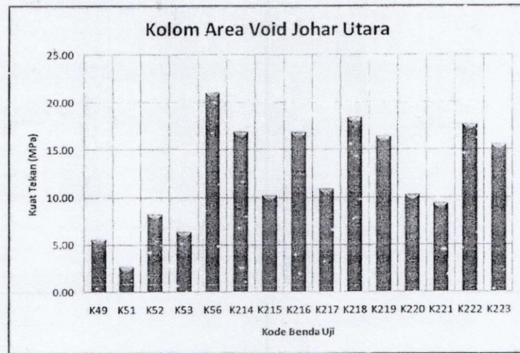
Gambar 18 Kurva sebaran nilai kuat tekan beton kolom area void Pasar Johar Utara
