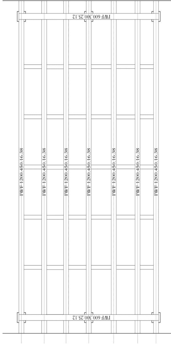
Gambar Profil Gelagar Memanjang dan Gelagar Melintang Skala 1:100
