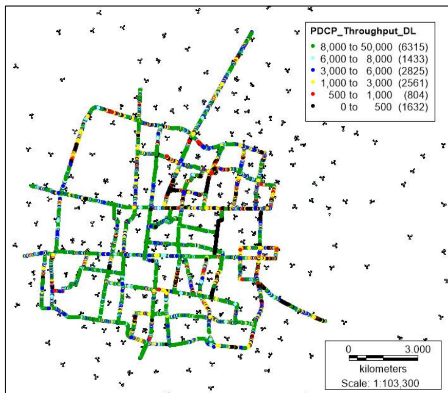
Gambar 16 Tampilan PDCP Throughput Download Data Plotting Februari 2018
