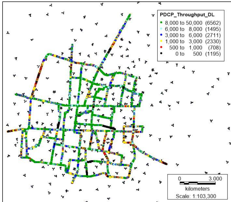
Gambar 15 Tampilan PDCP Throughput Download Data Plotting Januari 2018
