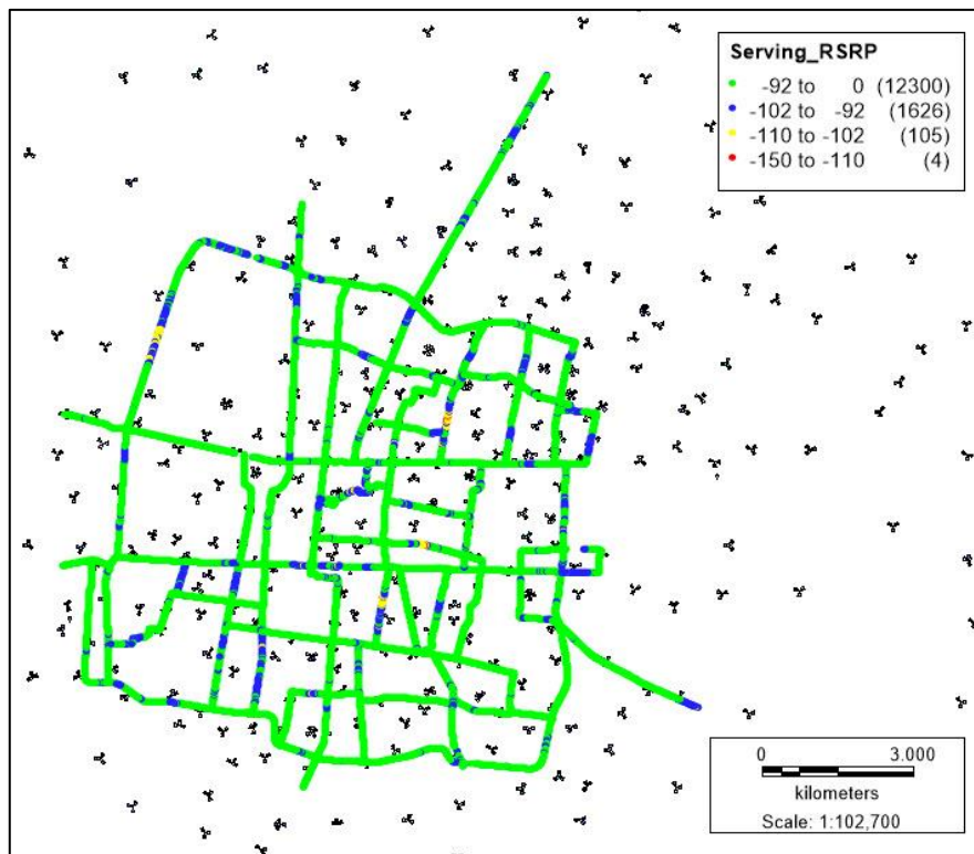
Gambar 7 Tampilan RSRP Data Plotting Juli 2018
