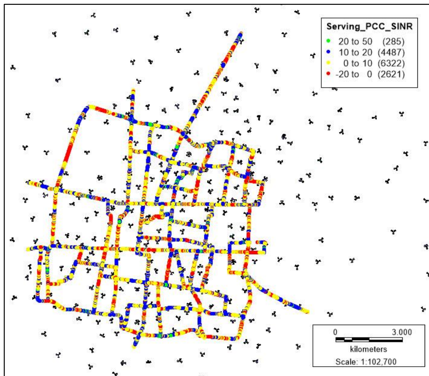
Gambar 14 Tampilan SINR Data Plotting Juli 2018
