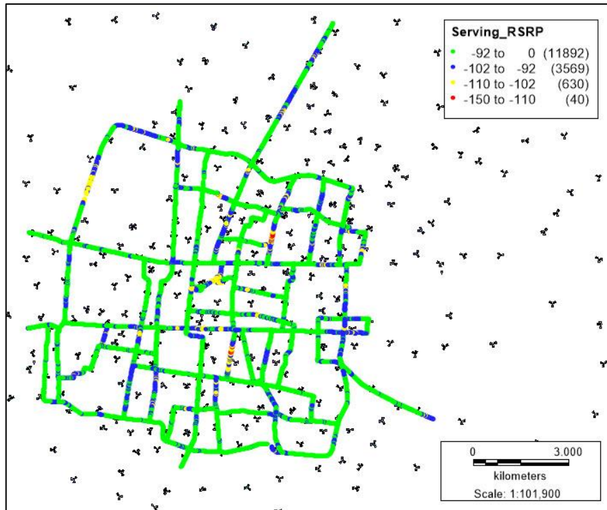
Gambar 5 Tampilan RSRP Data Plotting Mei 2018
