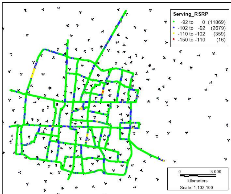
Gambar 6 Tampilan RSRP Data Plotting Juni 2018
