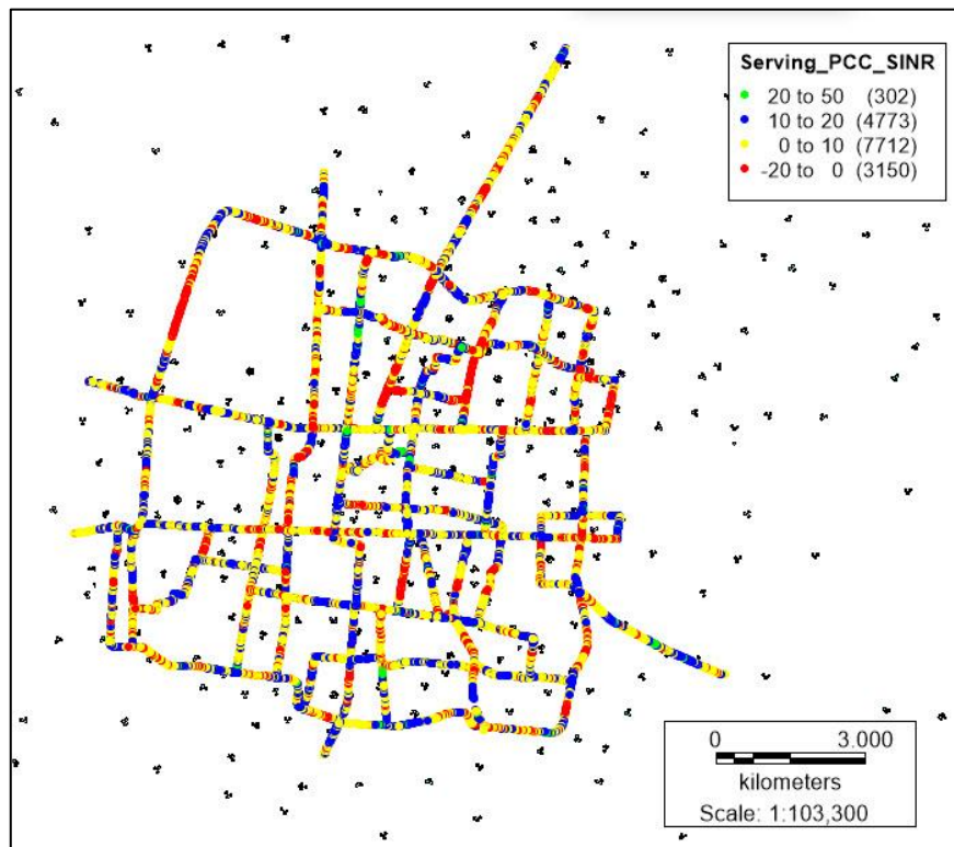
Gambar 9 Tampilan SINR Data Plotting Februari 2018
