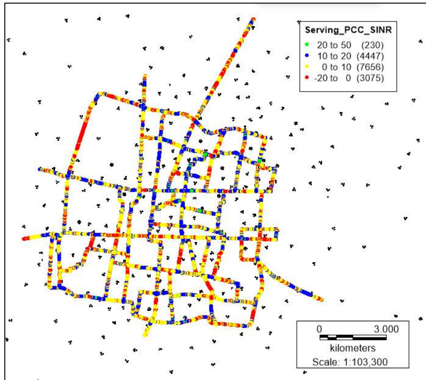
Gambar 8 Tampilan SINR Data Plotting Januari 2018
