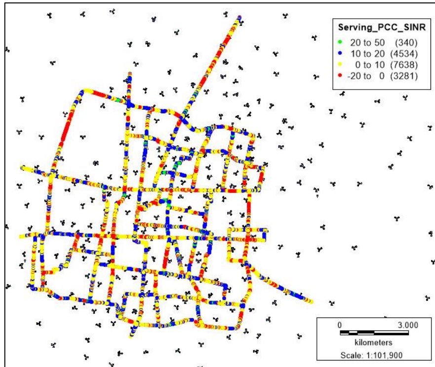
Gambar 12 Tampilan SINR Data Plotting Mei 2018
