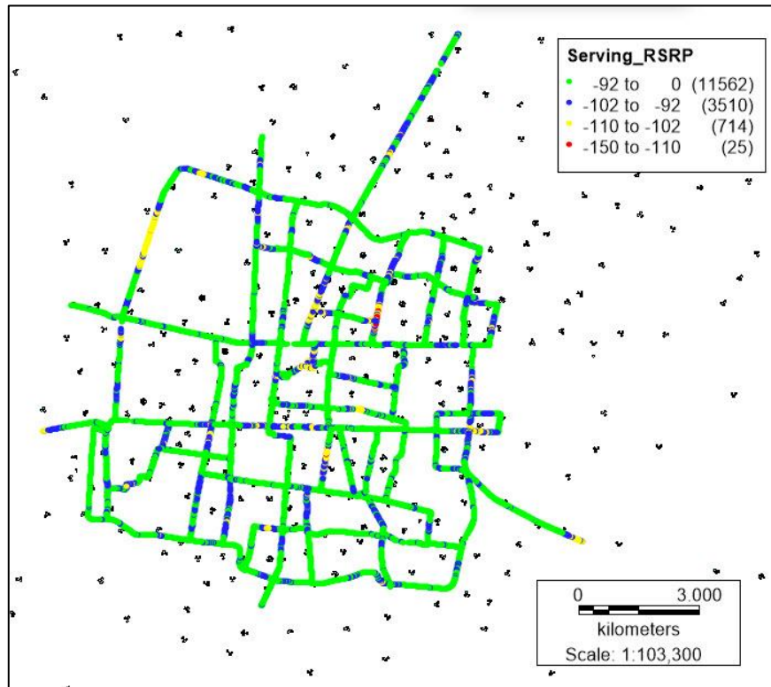
Gambar 1 Tampilan RSRP Data Plotting Januari 2018
