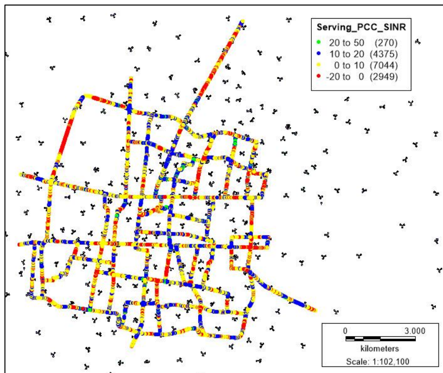
Gambar 13 Tampilan SINR Data Plotting Juni 2018
