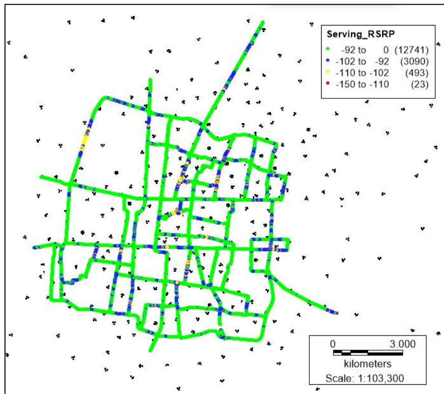
Gambar 2 Tampilan RSRP Data Plotting Februari 2018
