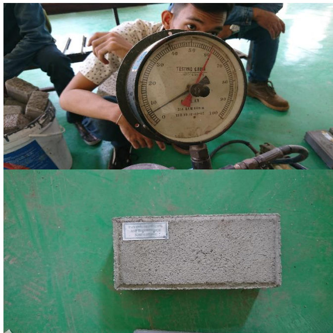
Gambar 18. Uji Kuat Lentur Cone Block ASP dan SKH 8%
