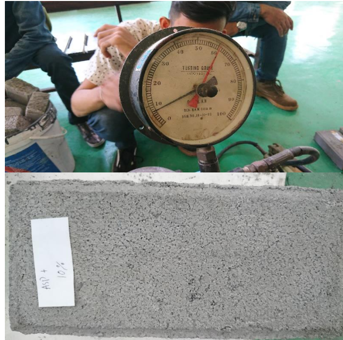
Gambar 37. Uji Kuat Lentur Cone Block Serbuk Kaca Hijau 10%
