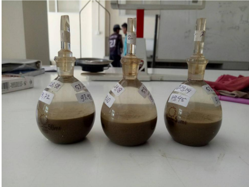
Pengujian Berat Jenis (Gs)
