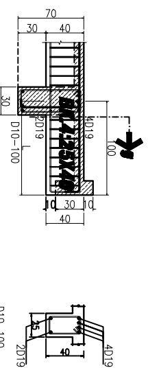
DETAIL BK.4 SKALA 1 : 40
