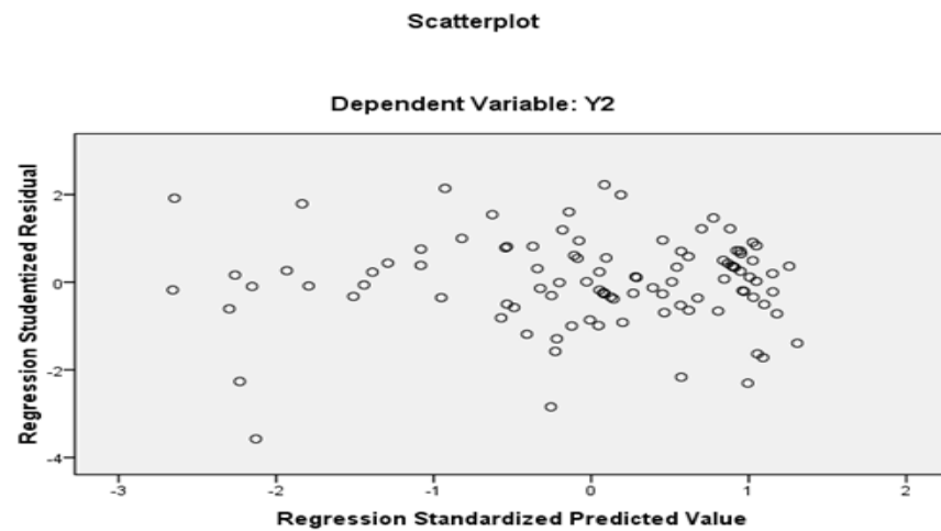
Gambar 4.2 Uji Heteroskedastisitas
