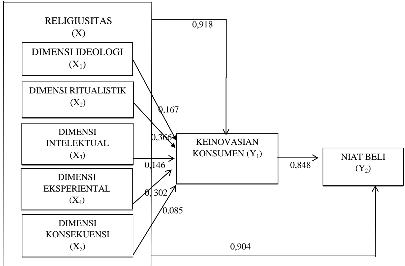
Gambar 4.3 Analisis Jalur
